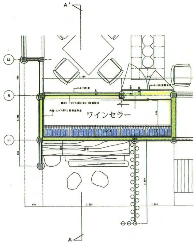
ワインセラー平面図
