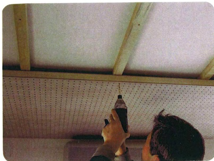
「隅のおさまり」
